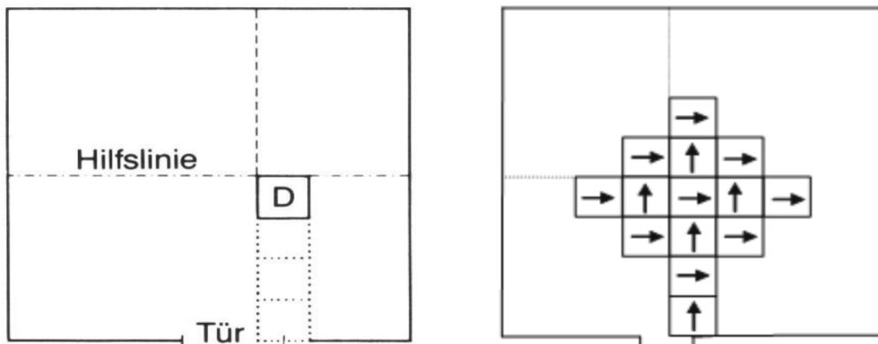
Anordnung der erste Fliesenreihe Parallel-/Schachbrett-Verlegung von Fliesen
